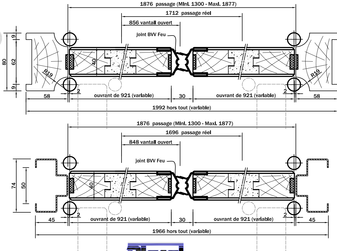
Plan de ferrage (voir chapitre 10)
